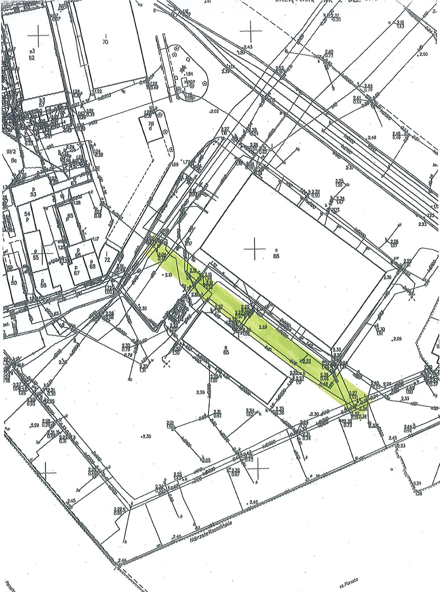
PRZYBLIŻONY PRZEBIEG RENOWOWANEJ SIECI WODOCIĄGOWEJ I KANALIZACYJNEJ
